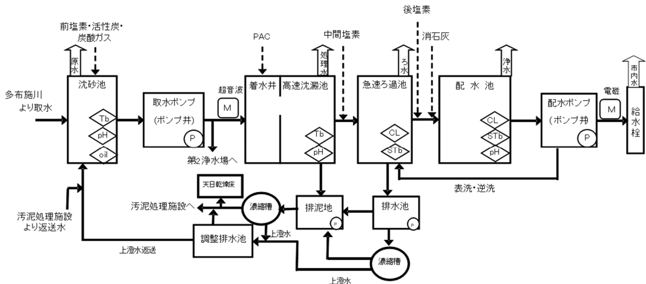
図-2 神野浄水場の処理工程図
