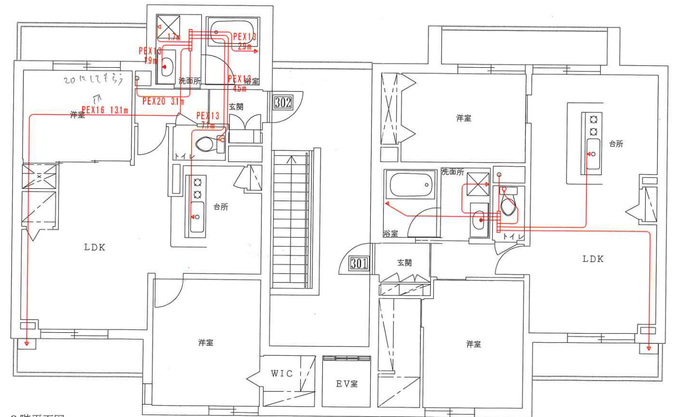
3階平面図
