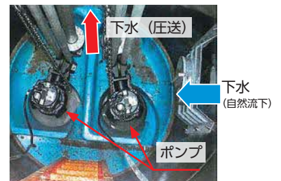
マンホールポンプ場内部
